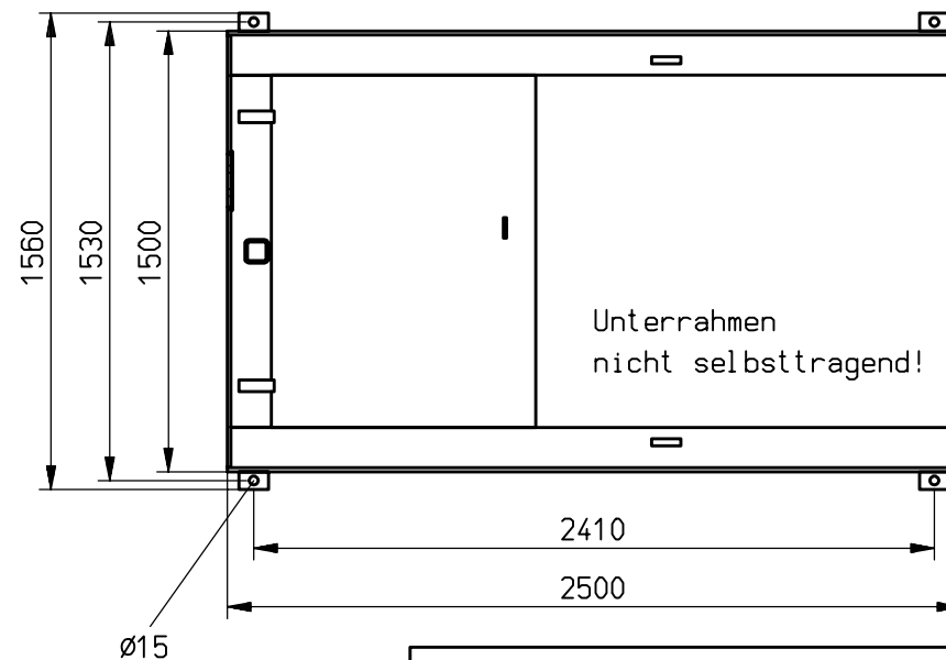
Maßblatt ELS 6-16-18
